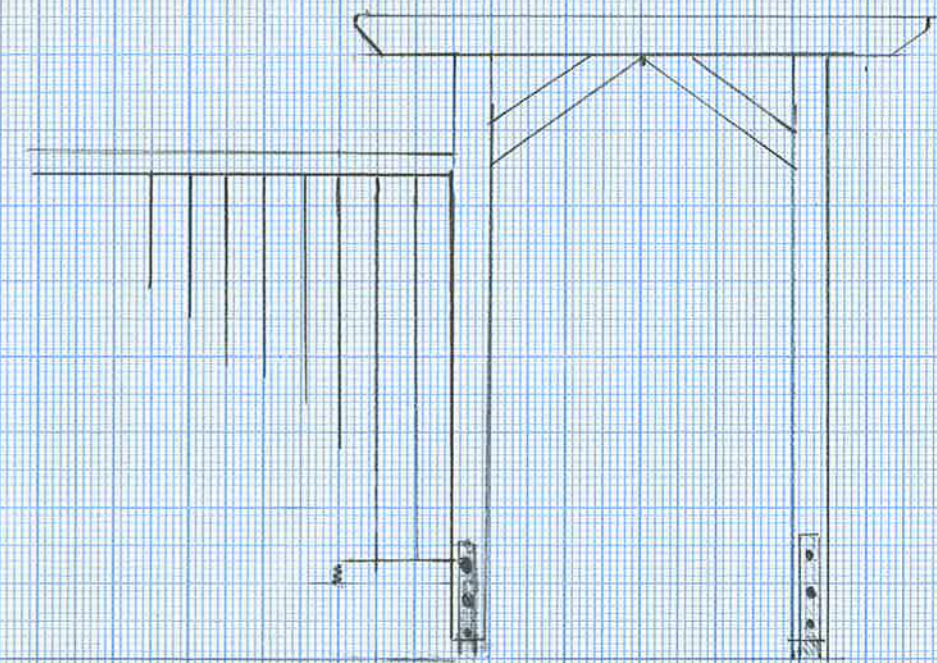
PORTAL SKALA 1:30
